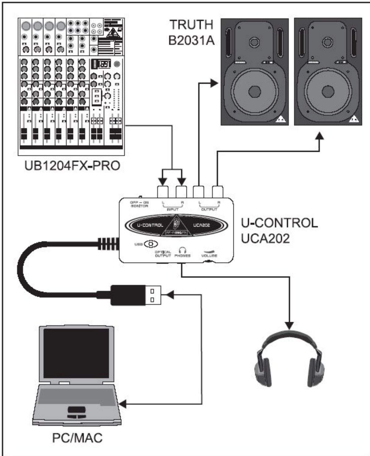
Exemple de système utilisant l'UCA202
